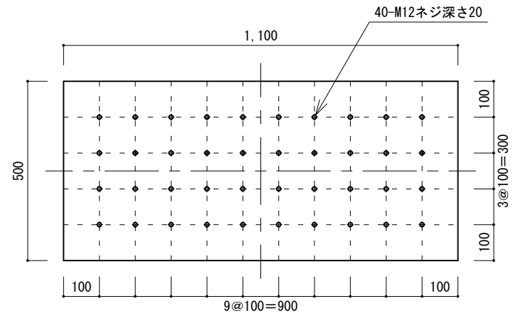
B 矢視
