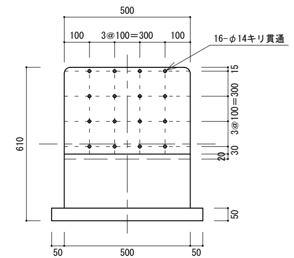
C 矢視
